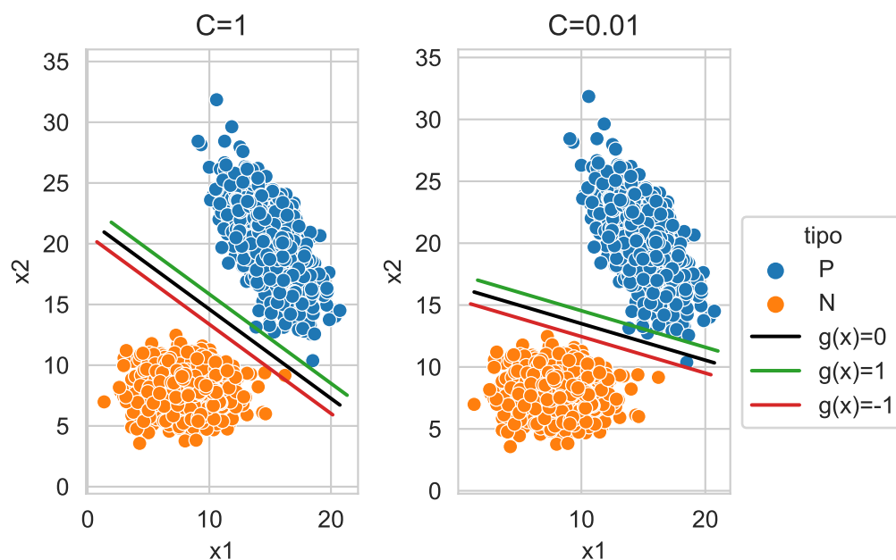
Figura 9.8: Hiperplanos para diferentes valores de C . Se observa que en C = 0.01 se clasifica incorrectamente un elemento positivo.
