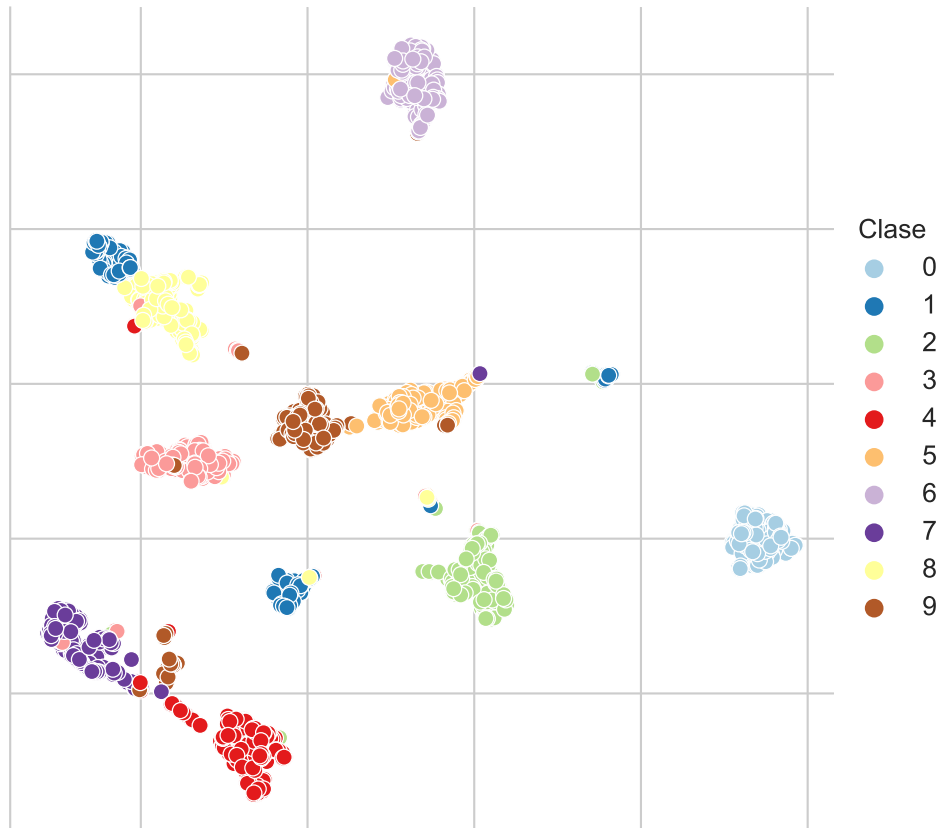
Figura C.5: Proyección mediante UMAP del problema de Dígitos con ocho vecinos.
