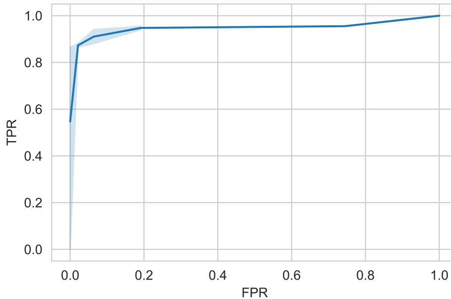
Figura 4.1: ROC
